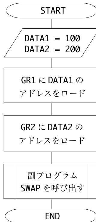
図1. 主プログラム MAIN のフローチャート
