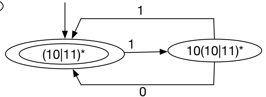
(d) (10|11)^*
