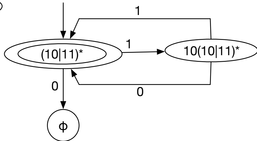
(d) (10|11)^*
