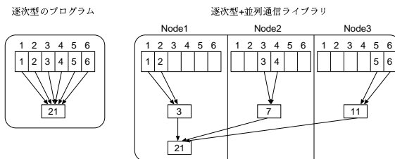
図 4 逐次型からの並列プログラミング Fig. 4 Parallel programming from sequential program
