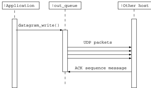
図 4 パケット送信時の動作を表すシーケンス図
