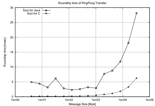
図 6 Suci for Java と C 言語版 Suci との比較 (ラウンドトリップタイム)
