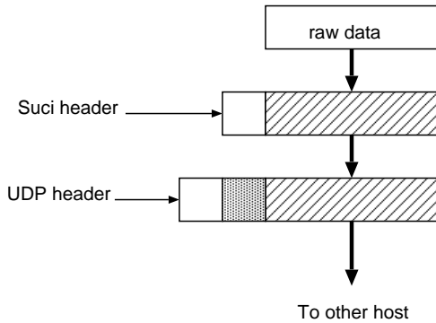
図 1 Suci と UDP スタックによるデータのカプセル化
