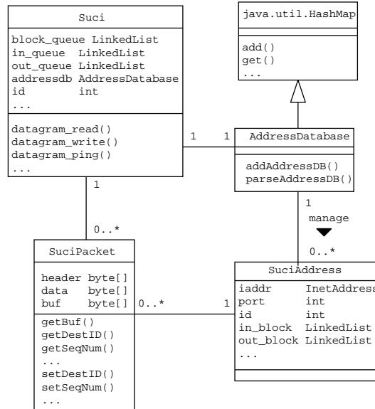
図 3 Suci for Java のクラス図
