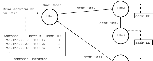
図 2 Suci による通信
