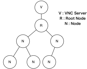
図 4 TreeVNC の構造
