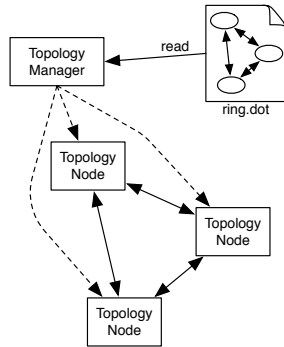
図 3 Topology Manager が記述に従いトポロジを構成
