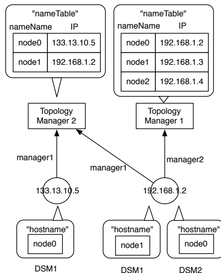
図 7 Topology Node は複数の nodeName を持つ
