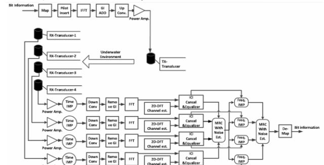
図 1 4 受信ダイバーシチシステムの送受信処理ブロック図
